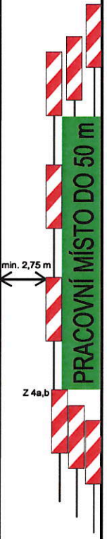
SCHÉMA B/2
